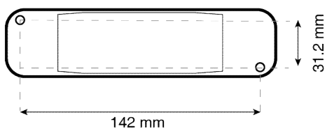
Abmessung der Montagelöcher
